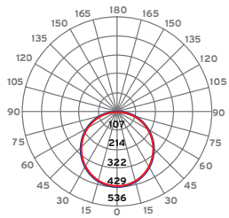
Curva de distribución de intensidad luminosa 18W
