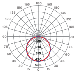
Curva de distribución de intensidad luminosa 18W Ángulo difuso promedio (50%): 115.3° — C0-C180 — C90-C270
